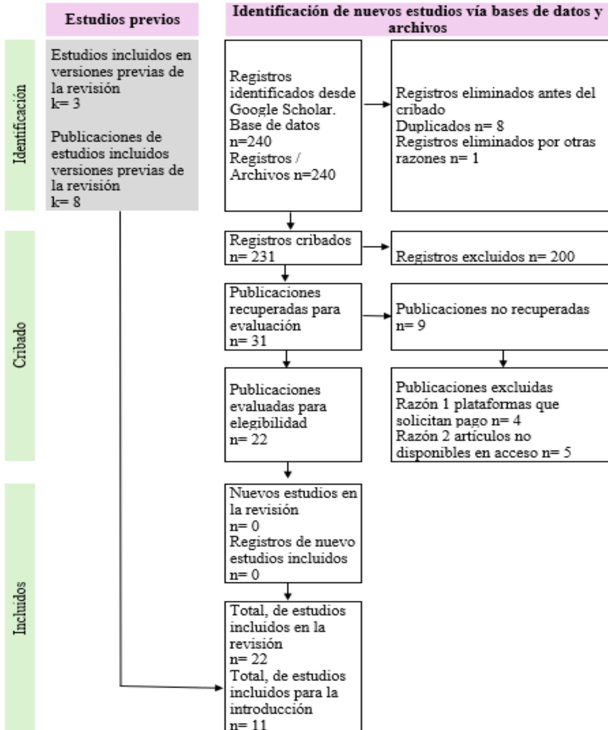
Figura 1. Esquema PRISMA
